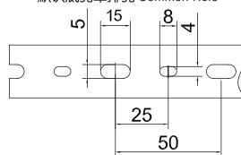
大小孔型号/Eu hole size: VDN4060F/614
