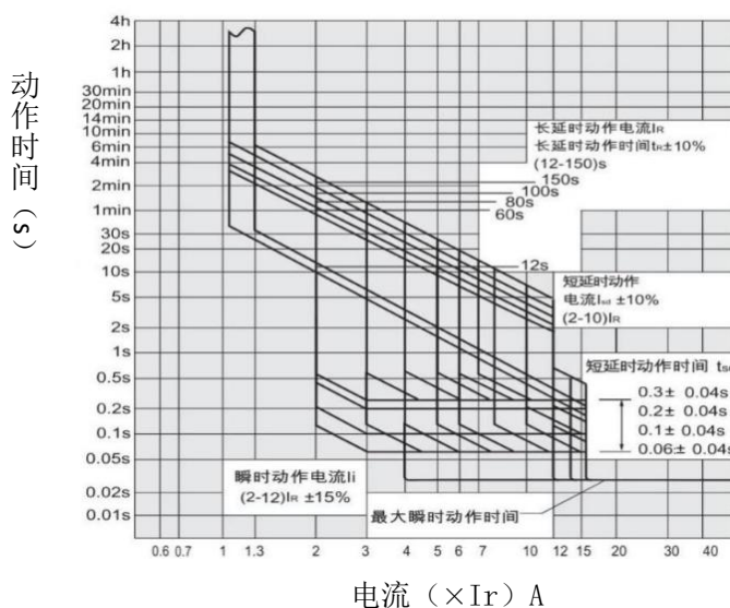
图 2 HYM3EP 系列塑料外壳式断路器特性曲线
