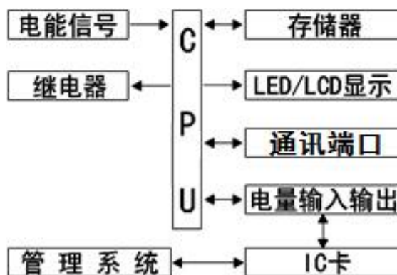
图2 电能表原理框图
