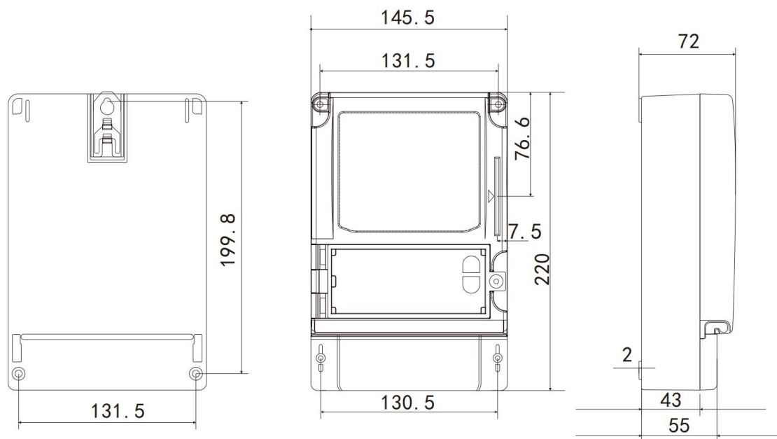
图5 DTSY6866 型电子式三相四线预付费电能表安装尺寸图
