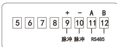
图4 功能端子接线图
