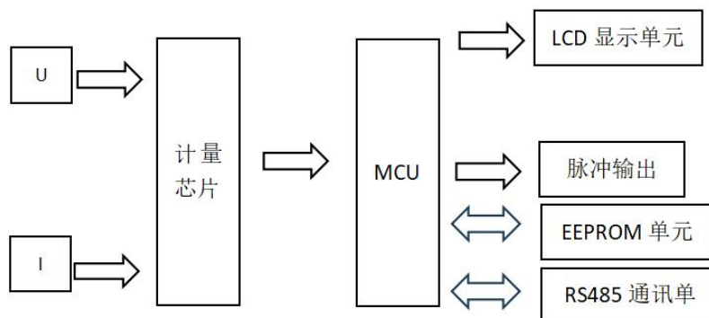
图2 工作原理图
