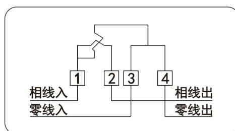
图3 接线图
