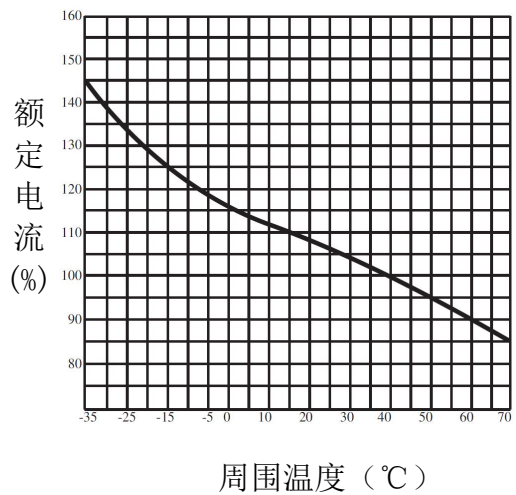
图2 HYM3-63 温度补偿曲线 HYM3-125 ≤63A 温度补偿曲线 HYM3-160 ≤63A 温度补偿曲线
