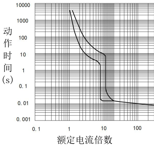
图1 HYM3-63 动作特性曲线 HYM3-125 ≤63A 动作特性曲线 HYM3-160 ≤63A 动作特性曲线
