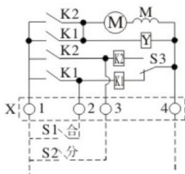
HYM1K-400、630、800、1250 电动操作机构分、合闸原理图
