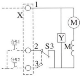
HYM1K-400、630、800、1250 电动操作机构分、合闸原理图
