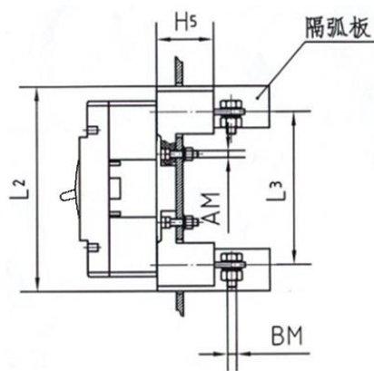
插入式接线
