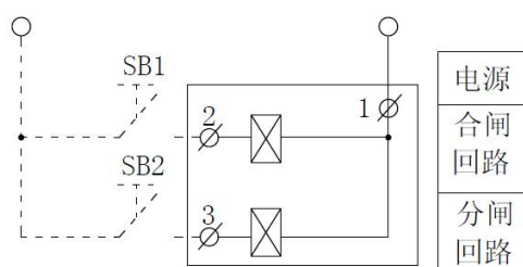
HYM1K-63、125、250 电动操作机构分、合闸原理图
