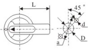
A 型(方形)手柄的外形及安装开孔
