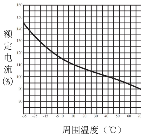
图 4 HYM3-125 >63A 温度补偿曲线
