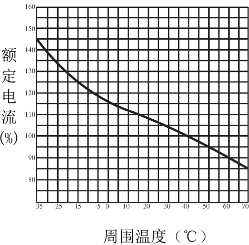
图 2 HYM3-63 温度补偿曲线
