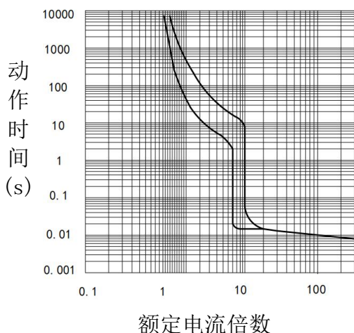
图 5 HYM3-160 >63A 动作特性曲线
