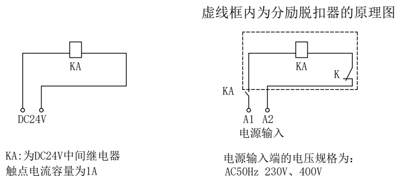
图 15 分励脱扣器控制回路设计
