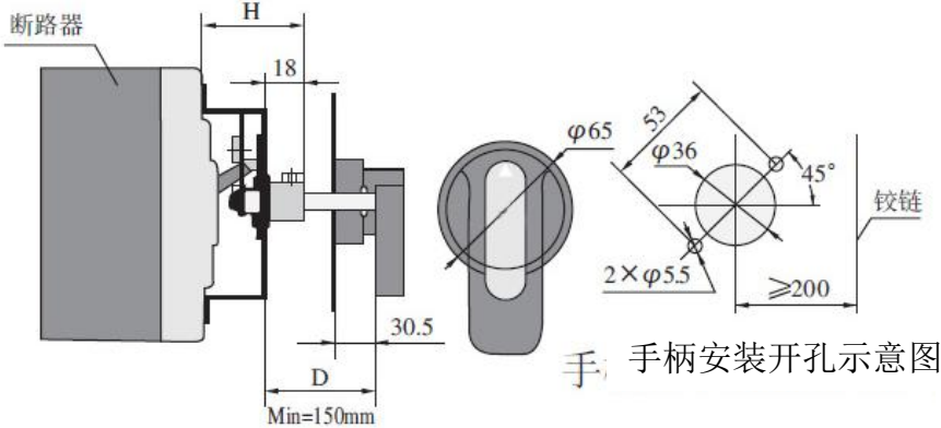
图 18 手动操作机构安装尺寸
