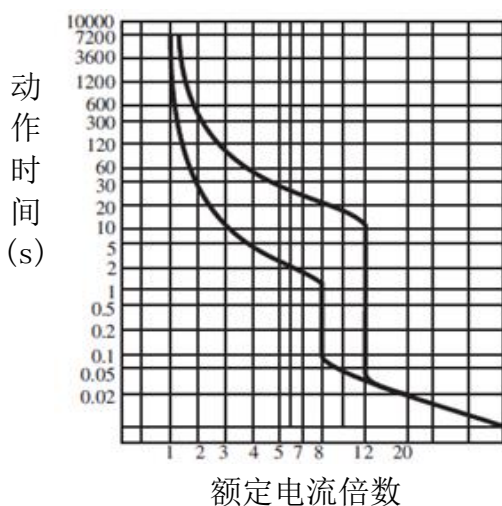
图 5 HYM3L-250 动作特性曲线
