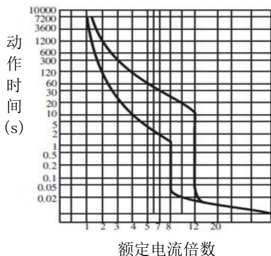
图 9 HYM3L-630 动作特性曲线
