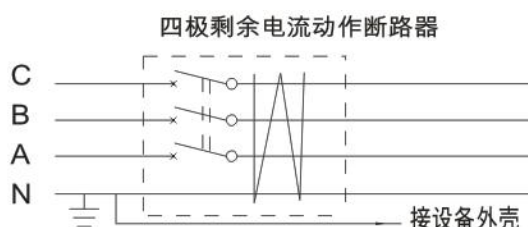
图 24 正确接线
