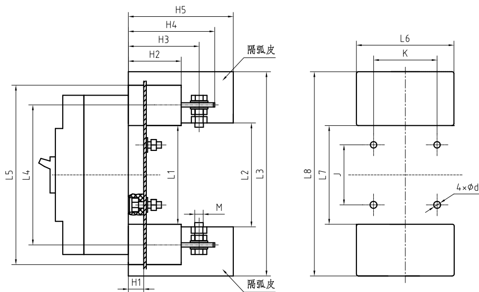
安装图
