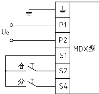
图 16 MDX 型电动操作机构的接线图
