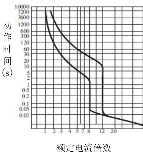
图 7 HYM3L-400 动作特性曲线
