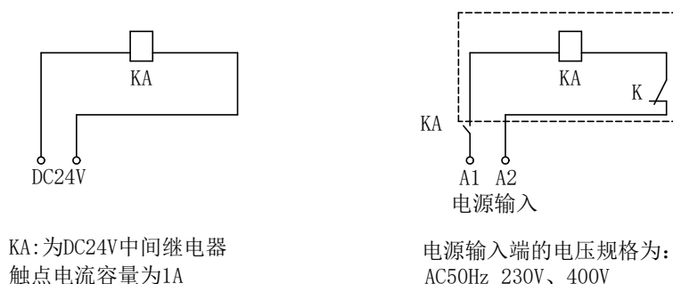
图 14 分励脱扣器控制回路设计
