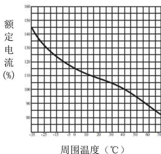
图 10 HYM3L-630 温度补偿曲线
