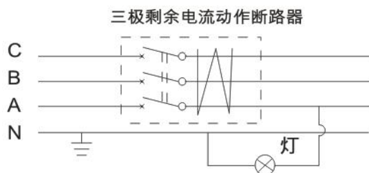
图 21 错误接线
