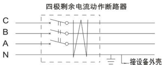
图 23 错误接线
