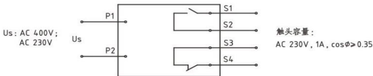
图 15 LB 型漏电报警模块接线图
