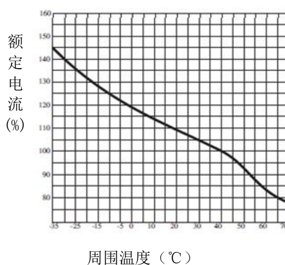
图 8 HYM3L-400 温度补偿曲线
