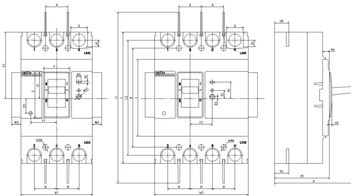
图 19 板前接线外形及安装尺寸
