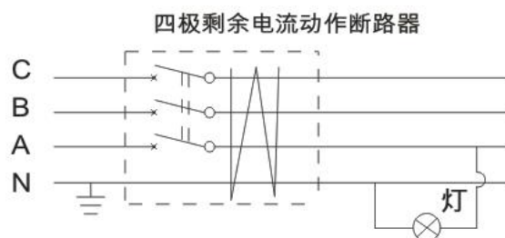
图 26 正确接线
