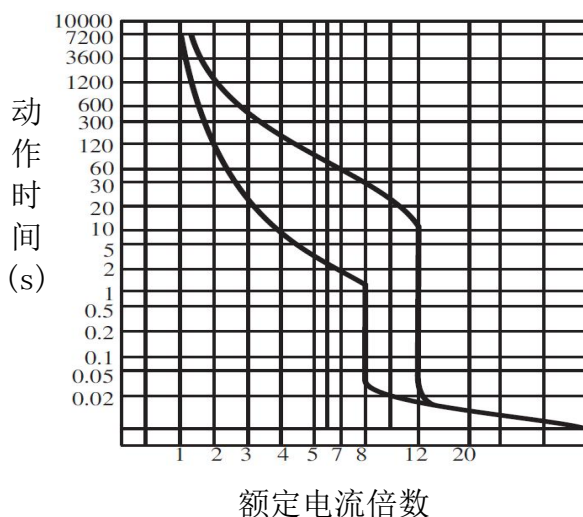
图 11 HYM3L-800 动作特性曲线
