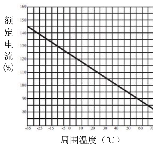
图 6 HYM3L-250 温度补偿曲线
