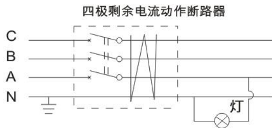
图 22 正确接线
