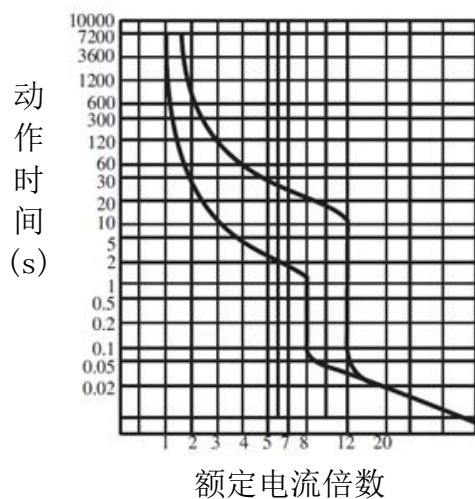
图 3 HYM3L-160 动作特性曲线
