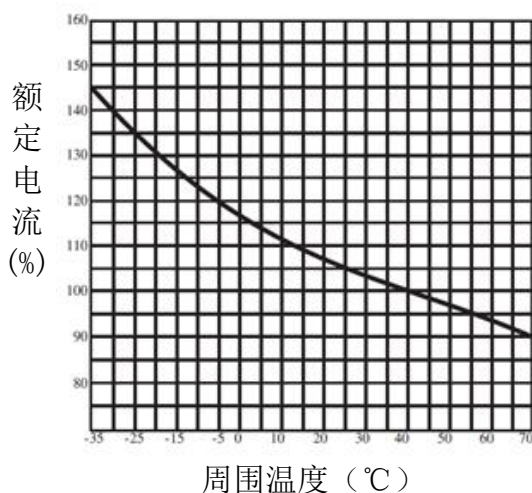
图 2 HYM3L-125 温度补偿曲线
