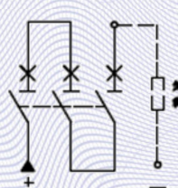
—— F型接线方式
