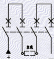
—— H型接线方式
