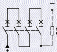
—— I型接线方式
