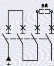
—— G型接线方式
