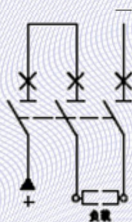
—— E型接线方式
