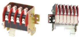
1000A壳架辅助开关
