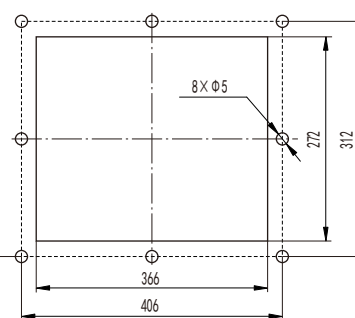
柜门开孔尺寸
