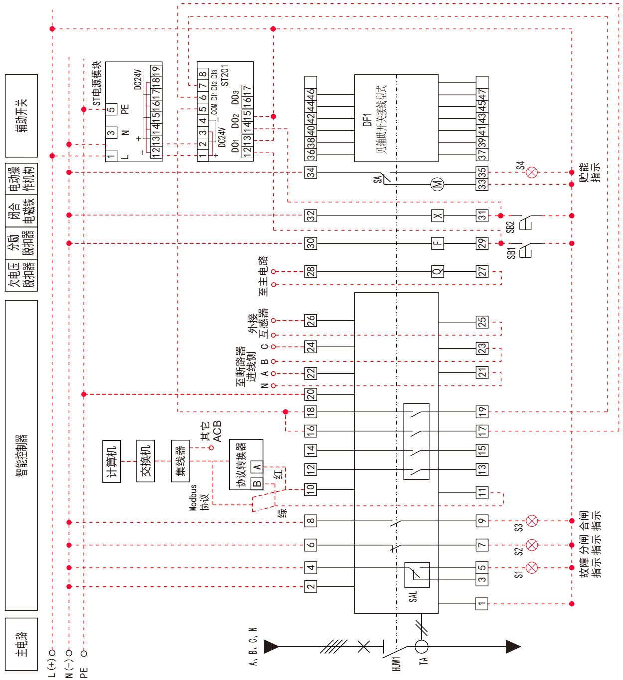
HUV1-2000及以上2H/3H型智能控制器二次回路接线图
