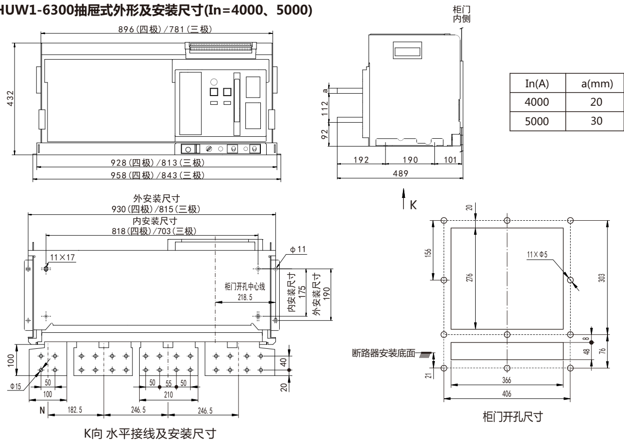
9.14 HUW1-6300抽屉式外形及安装尺寸(In=6300)
