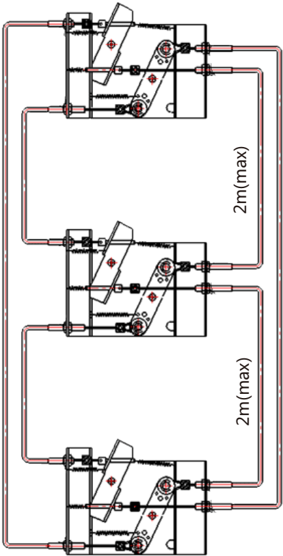
钢缆三联锁示意图
