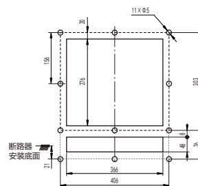
柜门开孔尺寸
