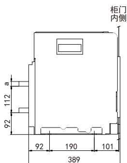
水平接线母排尺寸
