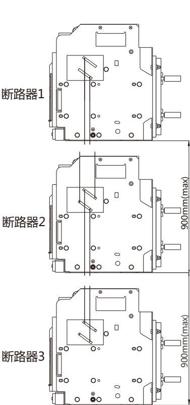
杠杆三联锁示意图
